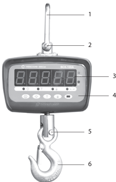
Рисунок 1. Весы ВСК-А.
